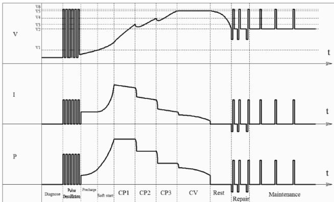
Figuur 3: Oplaadkarakteristiek voor lood-zuurbatterij
