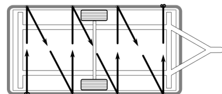
Afbeelding 2: Bevestiging met het spantouw
