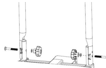
Bild 2: Montage U-Bügel
