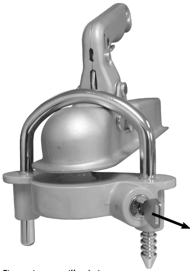
Figure 4 : verrouiller étrier
